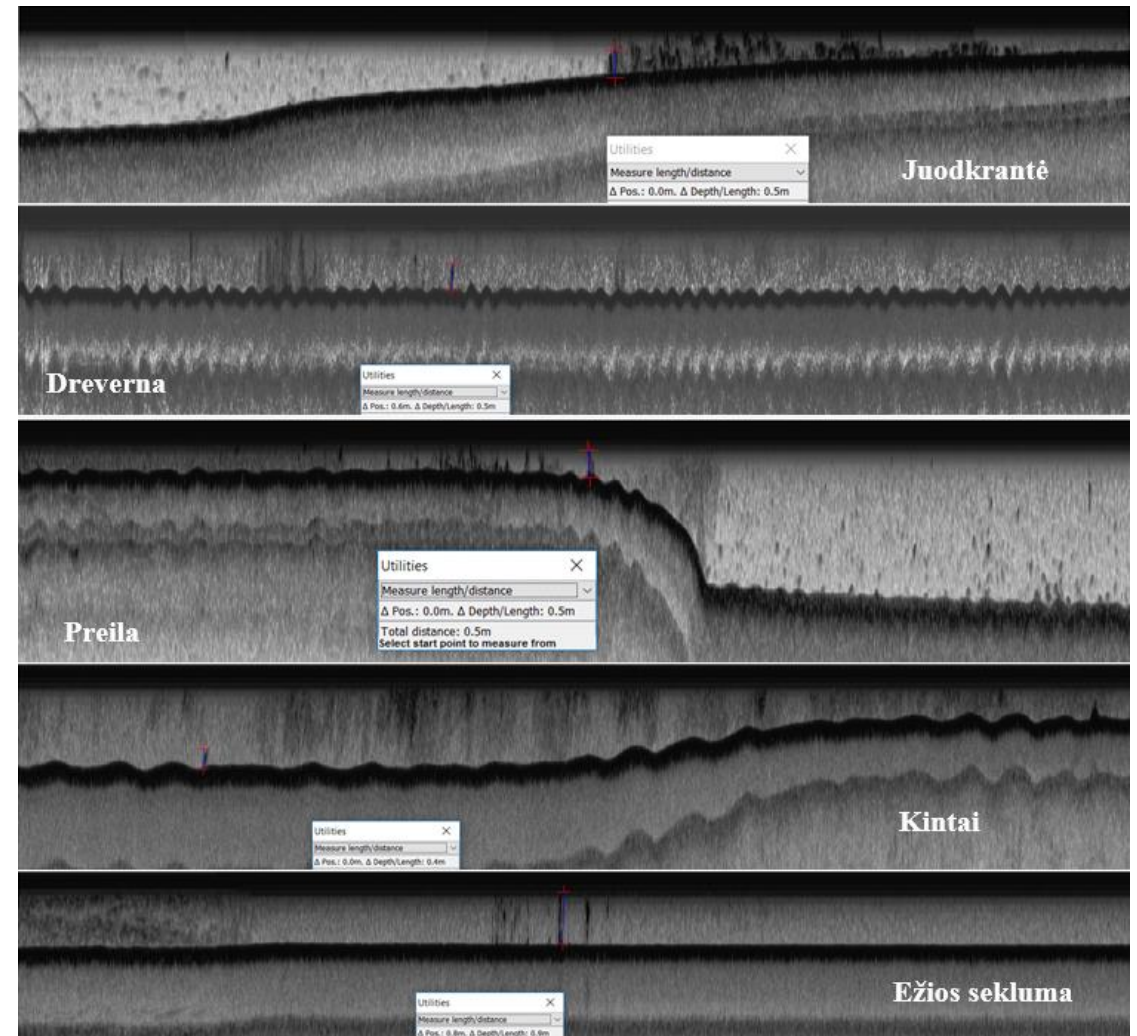
Sonaro echogramos
